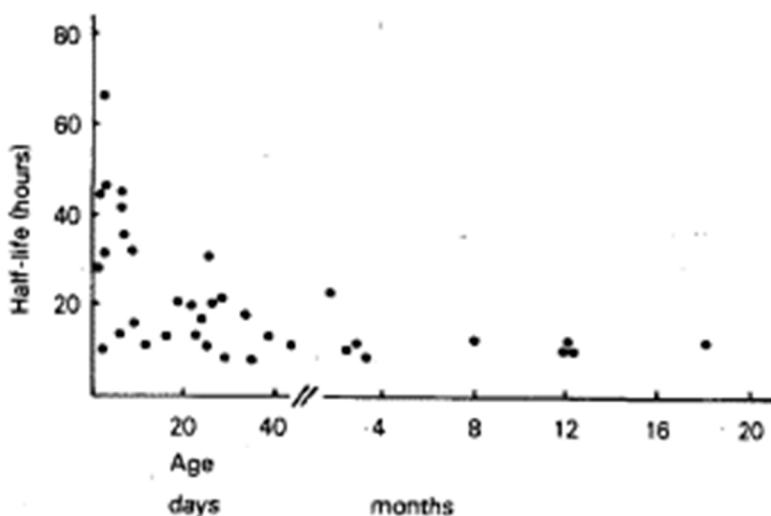
Figure 3 : Variation de la demi-vie selon l'âge chez le nourrisson jusqu'à 20 mois (Gugler et Von Unruh, 1980)
